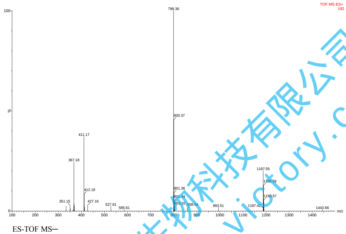
质谱MS图
